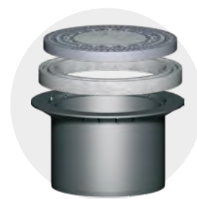
Teleskop pro poklop BEGU DN 600
